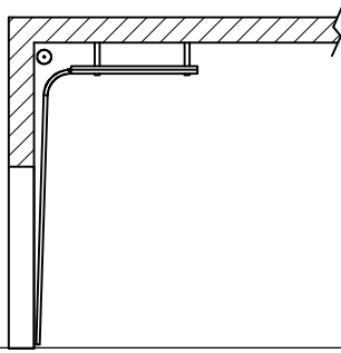
Installazione con guide prolungate
