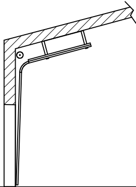
Installazione con guide prolungate su tetto inclinato
