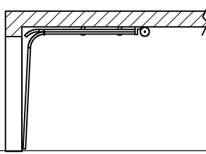
Installazione con architrave ridotto
