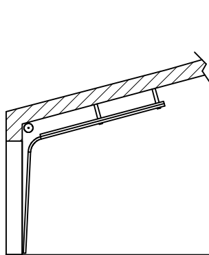
Installazione stanard su tetto inclinato
