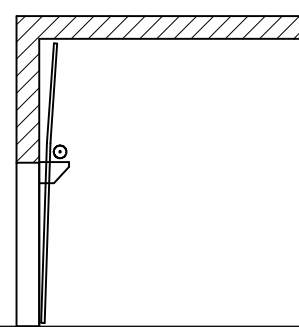
Installazione con albero portamolle ribassato
