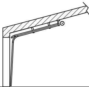
Installazione con architrave ridotto su tetto inclinato
